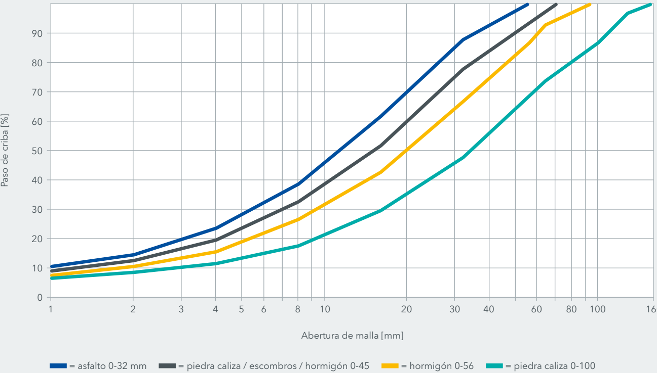
Curva de trituración MOBIREX - MR 110(i) EVO2 / MR 130(i) EVO2 en circuito abierto (< 15 % de fracción superior)
