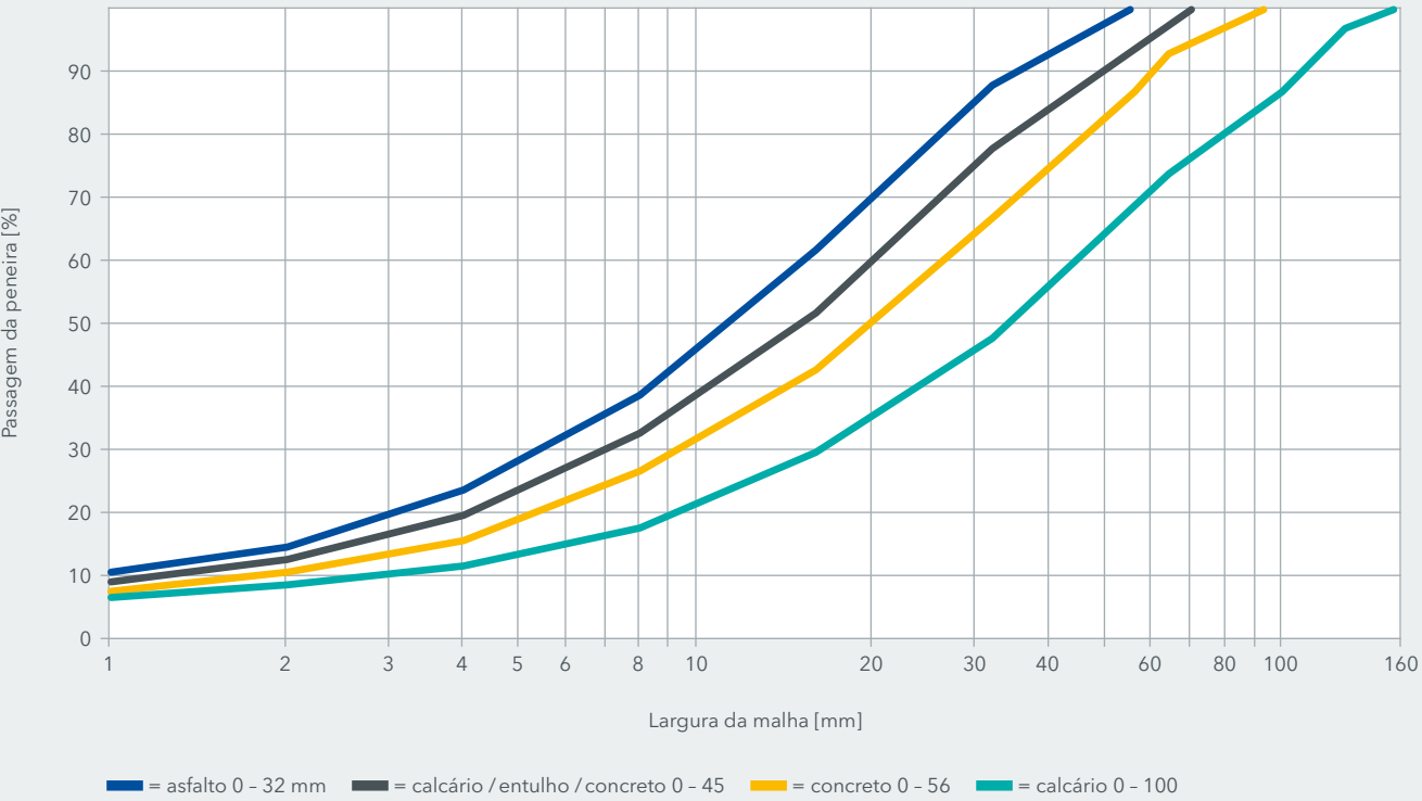
Curva de britagem MOBIREX - MR 110(i) EVO2 / MR 130(i) EVO2 no circuito aberto (< 15% de grânulo excessivamente grande)
